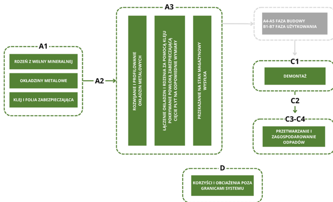
Rysunek 5.1: Granice systemu wykorzystane do charakterystyki środowiskowej
