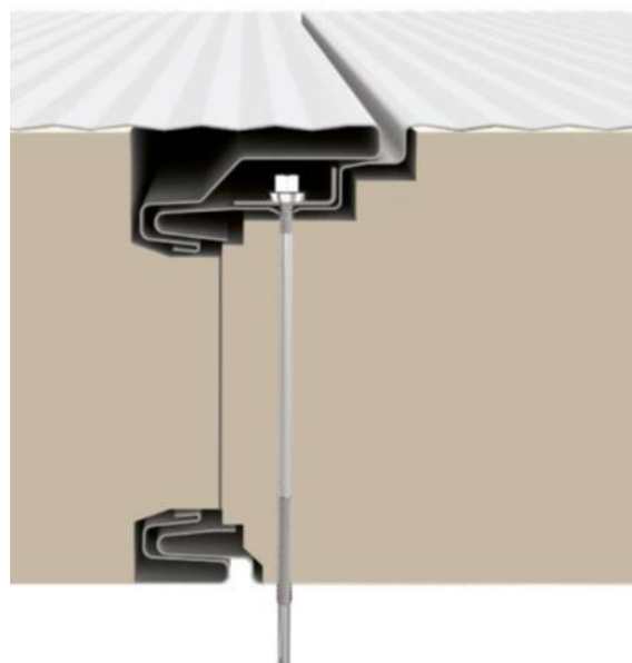
Rysunek 4.4: Przekrój płyty warstwowej IzoGold z rdzeniem z wełny mineralnej o zmiennej gęstości – ukryte mocowanie
